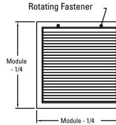
Face View (-6)
